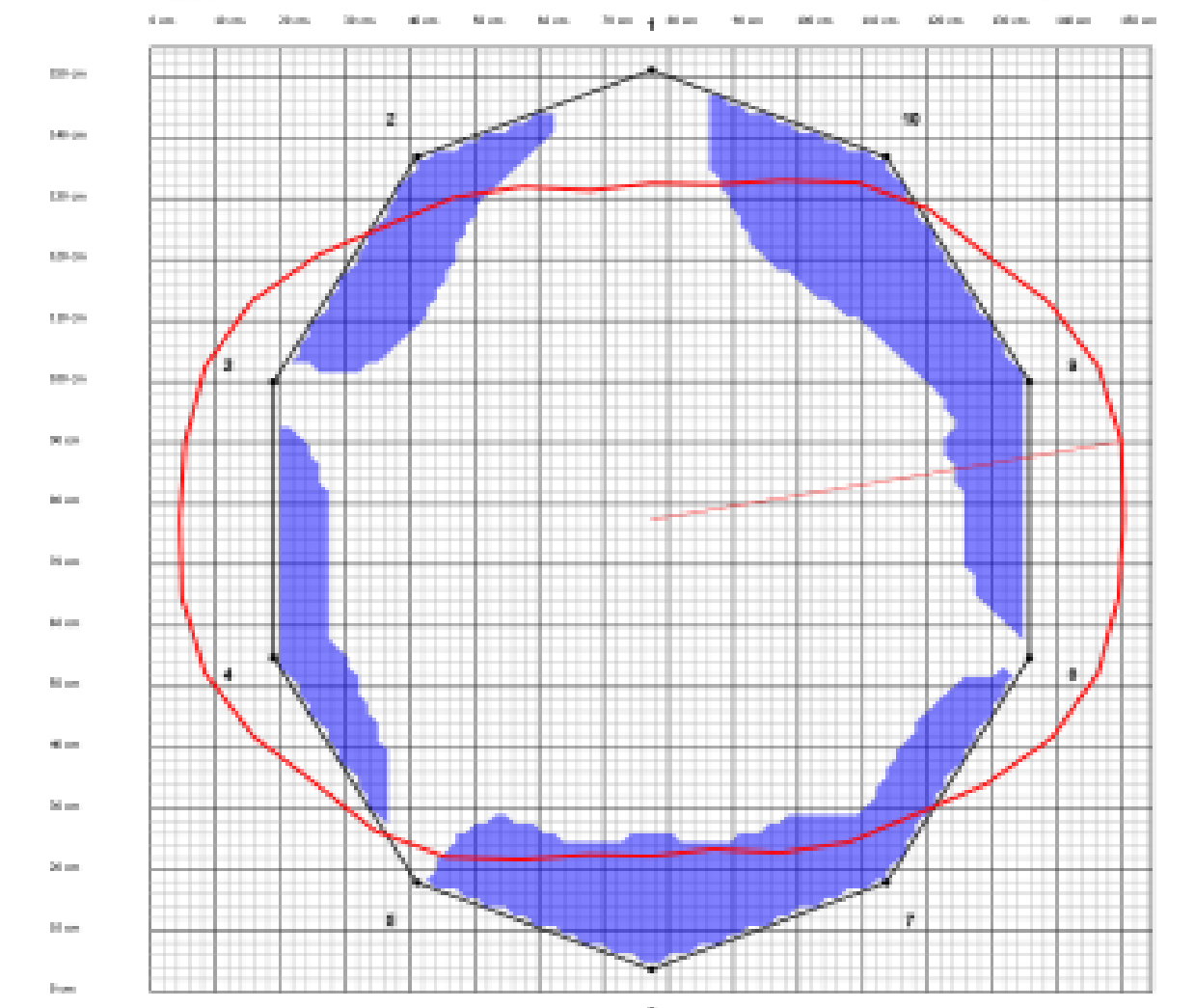
(2D a 3D tomogram poškodennej dreveny so zníženou stabilitou)
