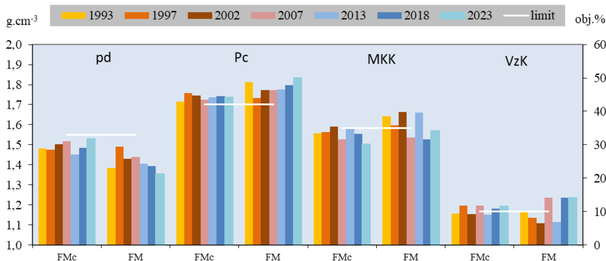
Obr. 3. Trend vývoja základných fyzikálnych vlastností podornice (0,30-0,40 m) piesočnato-hlinitých pôd. podľa pôdných typov a odberových cyklov
