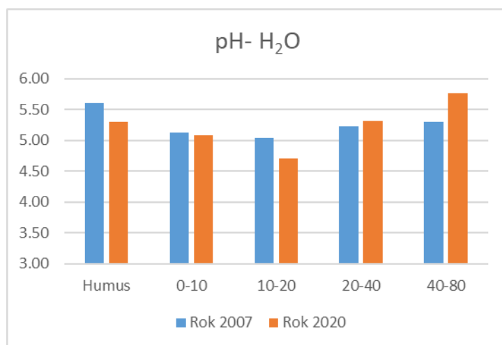
Obr. 3. Porovnanie nameraných hodnôt aktívnej reakcie v rokoch 2007 a 2020 podľa odberových hĺbok na TMP Čifáre
