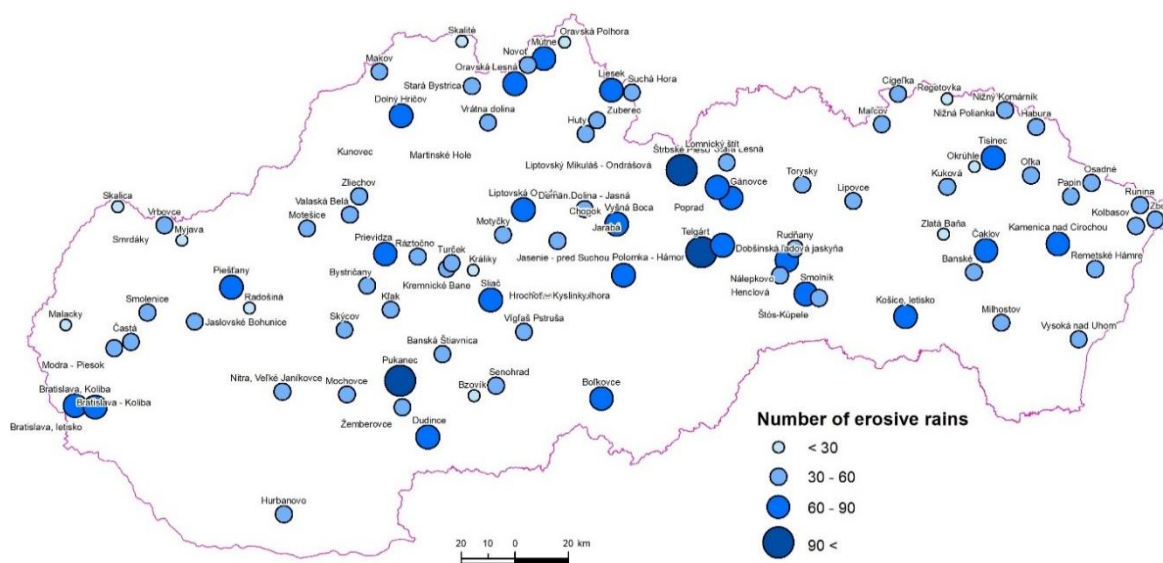
Obr. 2. Počty definovaných erózných účinných dažďov (za sledované obdobie) v rámci jednotlivých automatických zrážkových meracích staníc SHMU
