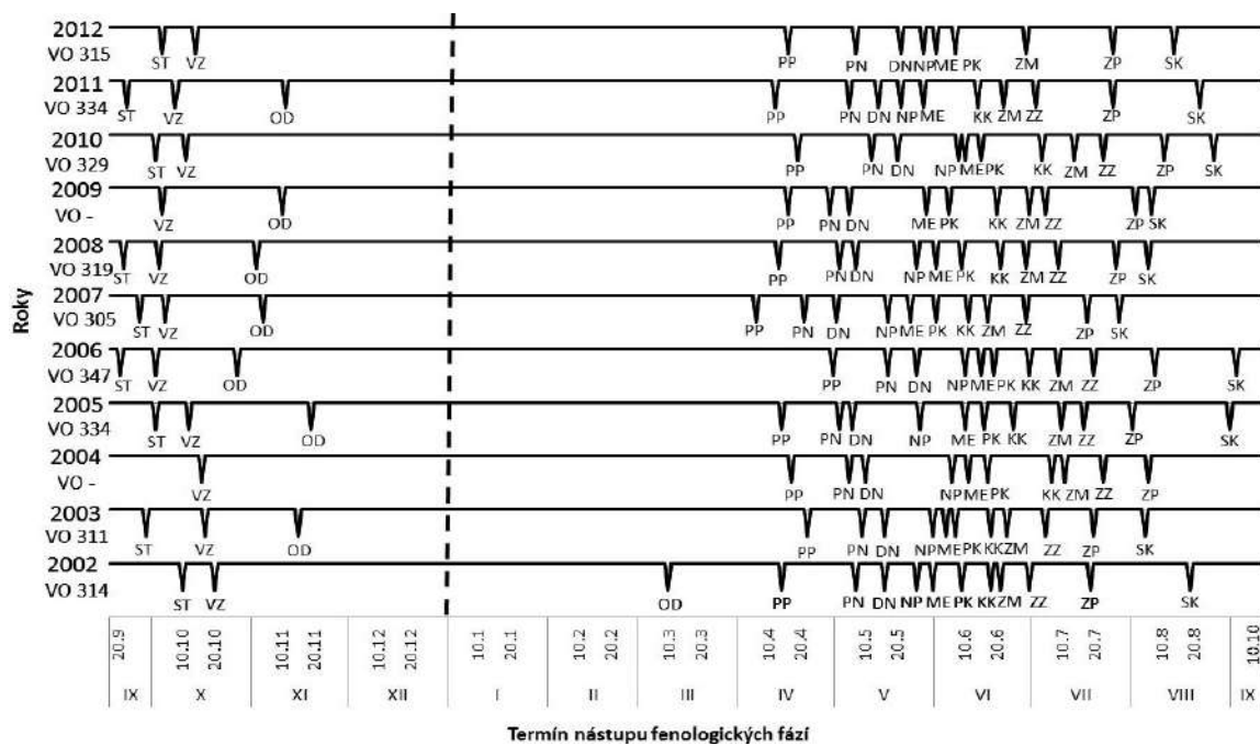
Graf 2: Nástup fenologických fází pšenice ozimé v období 2002–2012 (zkratky viz Materiál a Metodika).
